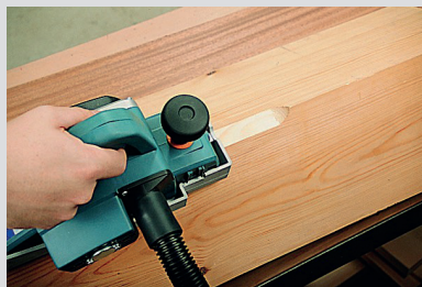
Verbindung zur Staubabsaugung mit dem Standard-Staubabsaugschlauch.
