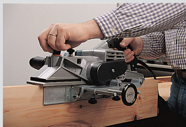
Verstellbarer Anschlag für verschiedene Fasen und Fasenwinkel.
