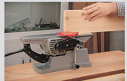
Stationäreinrichtung.
