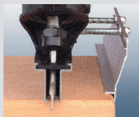
Fräsen mit Seitenanschlag
