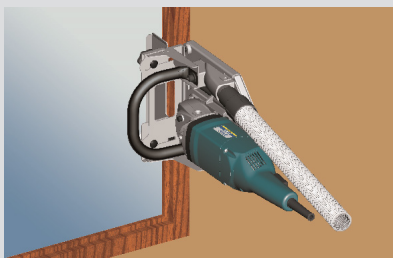
Heraustrennen des Rahmens durch einen sauberen, geführten Schnitt.
