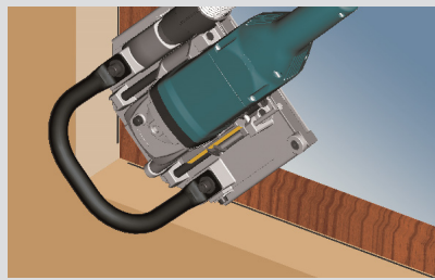
Komplettes Heraustrennen bis in die Ecke.
