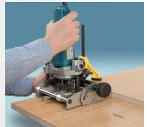
Fresado a 0°
